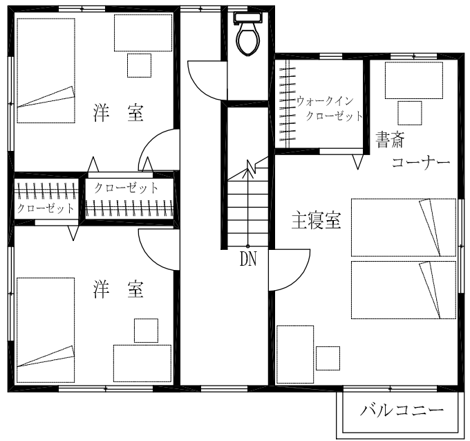
2階平面図
